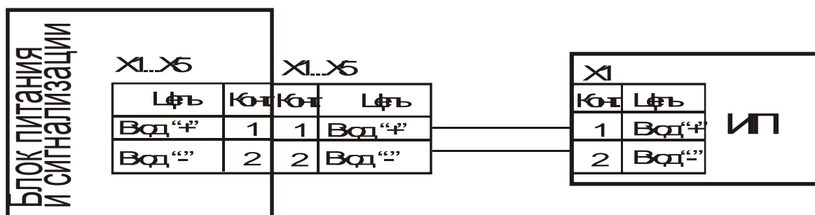
а) Схема подключения ИП-NH 3 :
