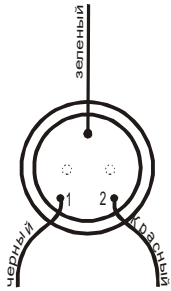
Рисунок 3 – Чувствительный элемент Sensor E-3. Схема распайки выводов
