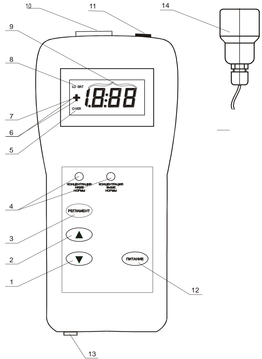
Рисунок 1 – Расположение органов управления, индикации и сигнализации
