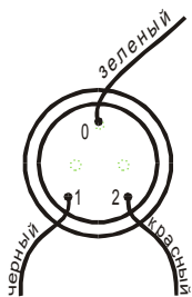
Рис. 3 – Чувствительный элемент Sensor E-3. Схема распайки выводов
